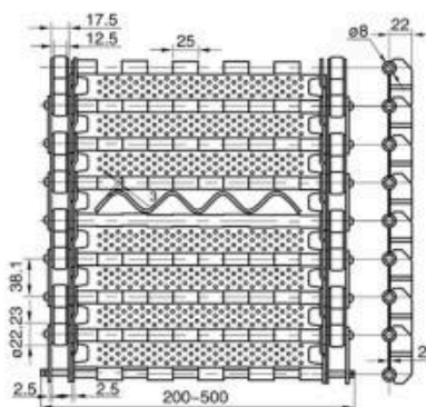
型号/Type: LJ:38.1mm (节距/pitch: 38.1mm)
