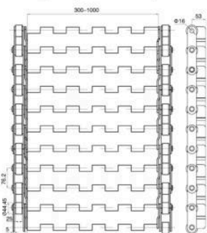
型号/Type: LJ:76.2mm (节距/pitch: 76.2mm)
