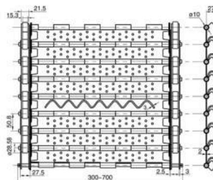
型号/Type: LJ:50.8mm (节距/pitch: 50.8mm)
